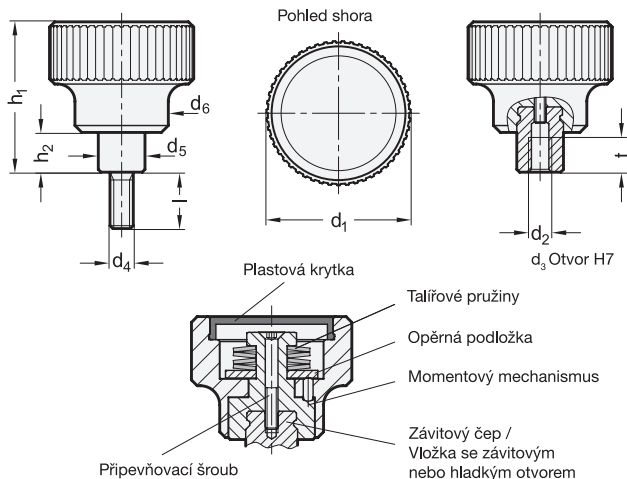
GN 3663-se závitovým čepem
